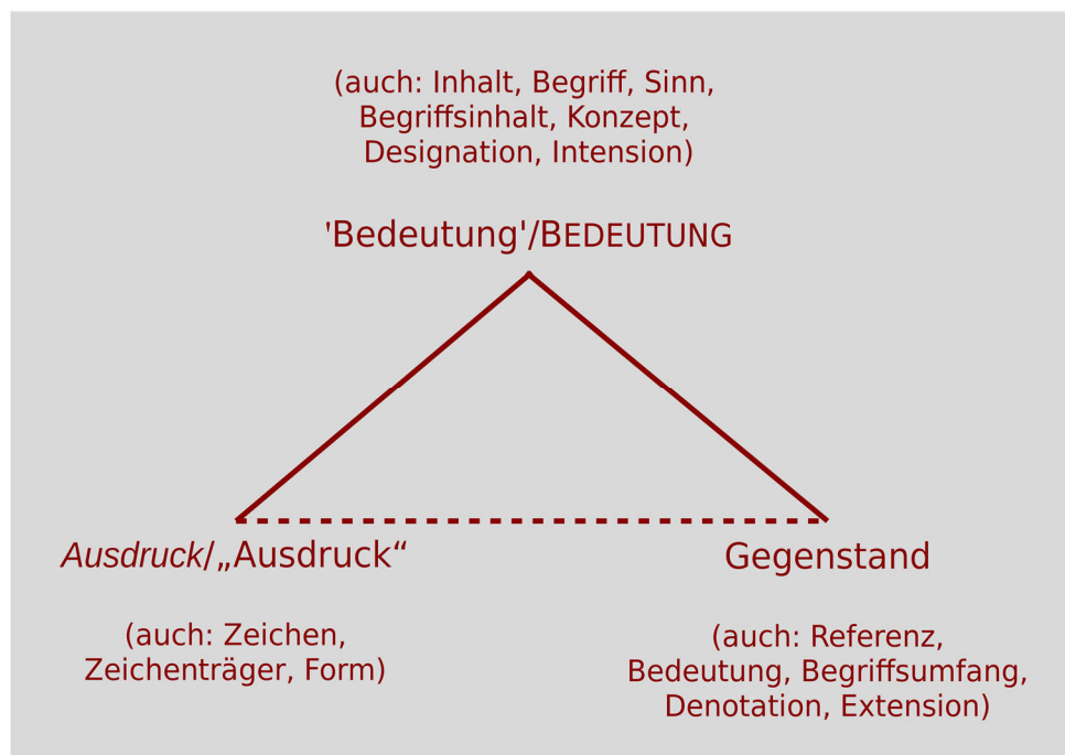
Semiotisches Dreieck
