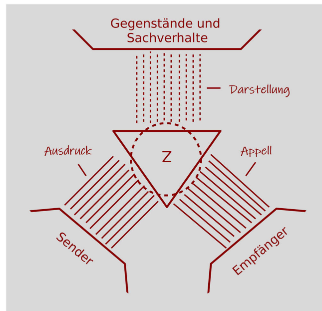
Organonmodell
