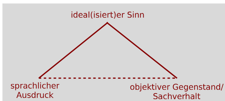
Freges Bedeutungskonzeption
